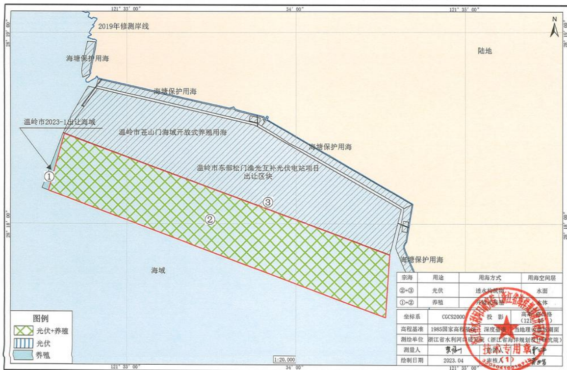
附件2：温岭市东部石塘渔光互补光伏电站项目转让区块宗海平面布置图
